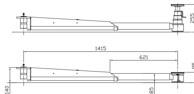
Long arm
